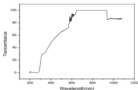
Fig. 2b UV-visible Spectra
