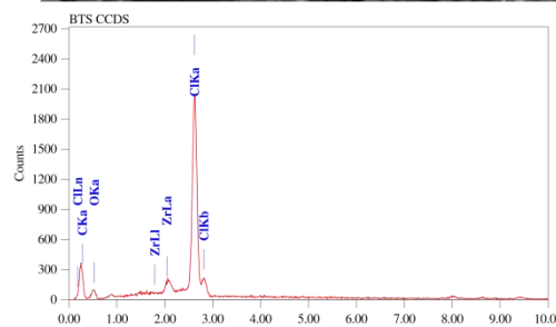
Fig. 3 EDAX Spectra
