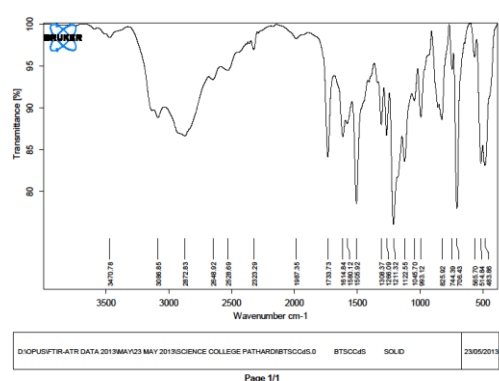
Fig. 1 FTIR Spectra
