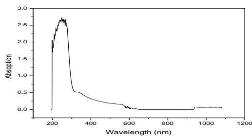
Fig. 2a. UV-visible Spectra
